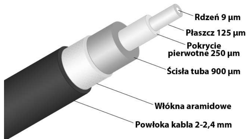
Rys. 1 Budowa światłowodu [3]
